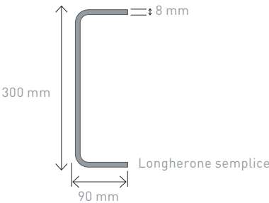
Telaio Heavy
