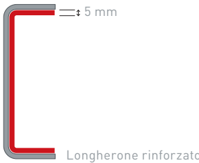
Telaio Xtrem
